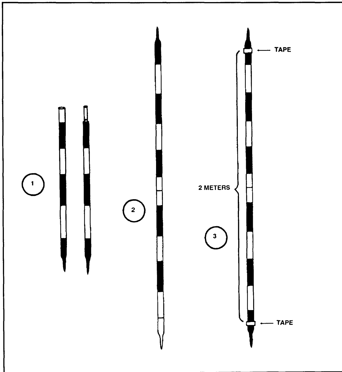
Figure C-7. Subtense bar.
